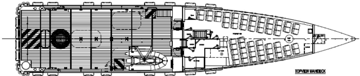
TOPVIEW MAINDECK
